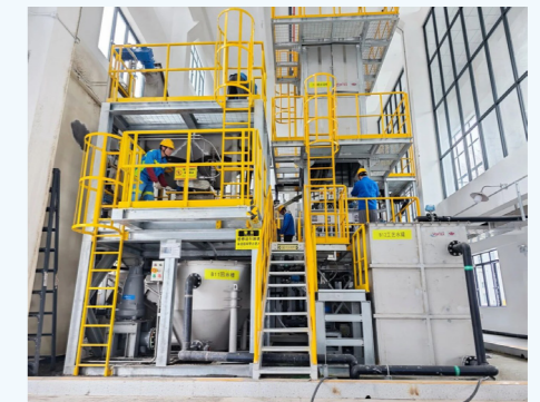
瀚蓝通沟污泥项目生产设备
